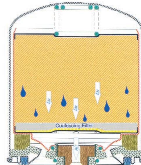
Koaleszenz-Effekt: Verbesserte Abscheidung kleinster Öltröpfchen (Aerosole)
